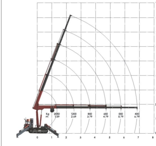
Lastdiagramm
