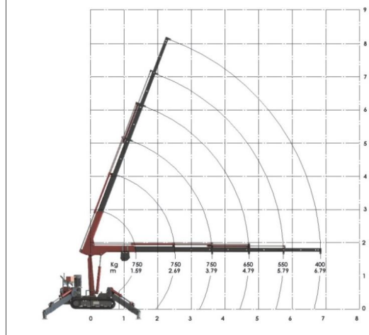
Lastdiagramm mit Winde
